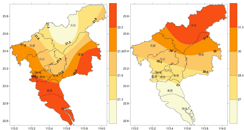
图 1 2025 年 11 月 3 日-11 月 9 日广州市平均气温（℃）和累计日照时数（小时）分布图
